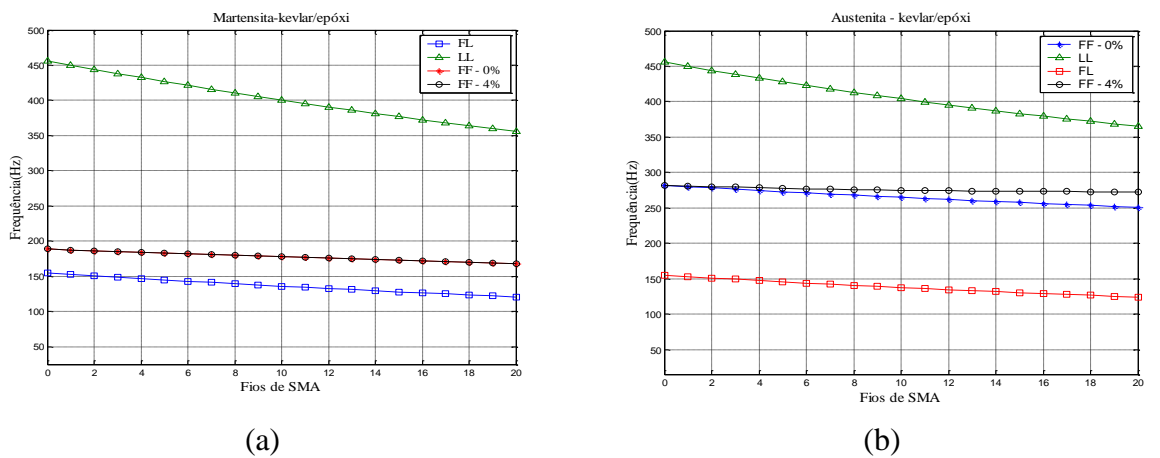
Figura 4. \omega_n em função de n para Epóxi/Fibra de kevlar sob as diferentes condições de contorno. a) Na fase martensita. b) Na fase austenítica.
