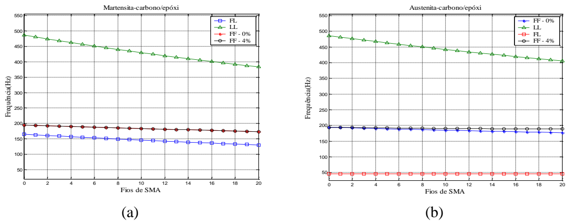
Figura 3. \omega_n em função de n para o compósito Epóxi/Fibra de carbono sob as diferentes condições de contorno. a) Na fase martensita. b) Na fase austenítica.
