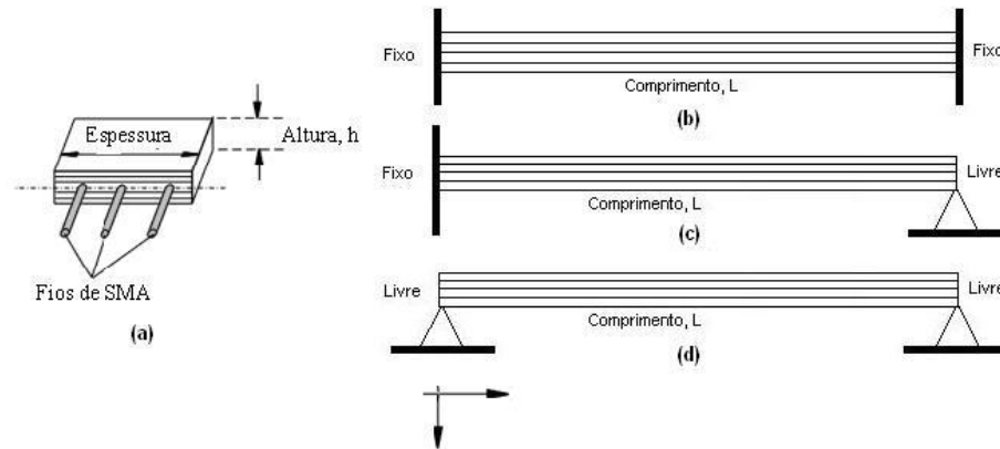
Figura 1. a) Viga compósita com fios de SMA embebidos. b) CC FF, c) CC FL). d) CC LL.
