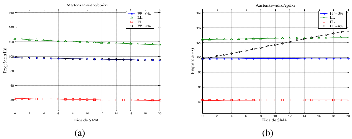
Figura 2. \omega_n em função de n para Epóxi/Fibra de vidro sob as diferentes condições de contorno. a) Na fase martensita. b) Fase austenítica.
